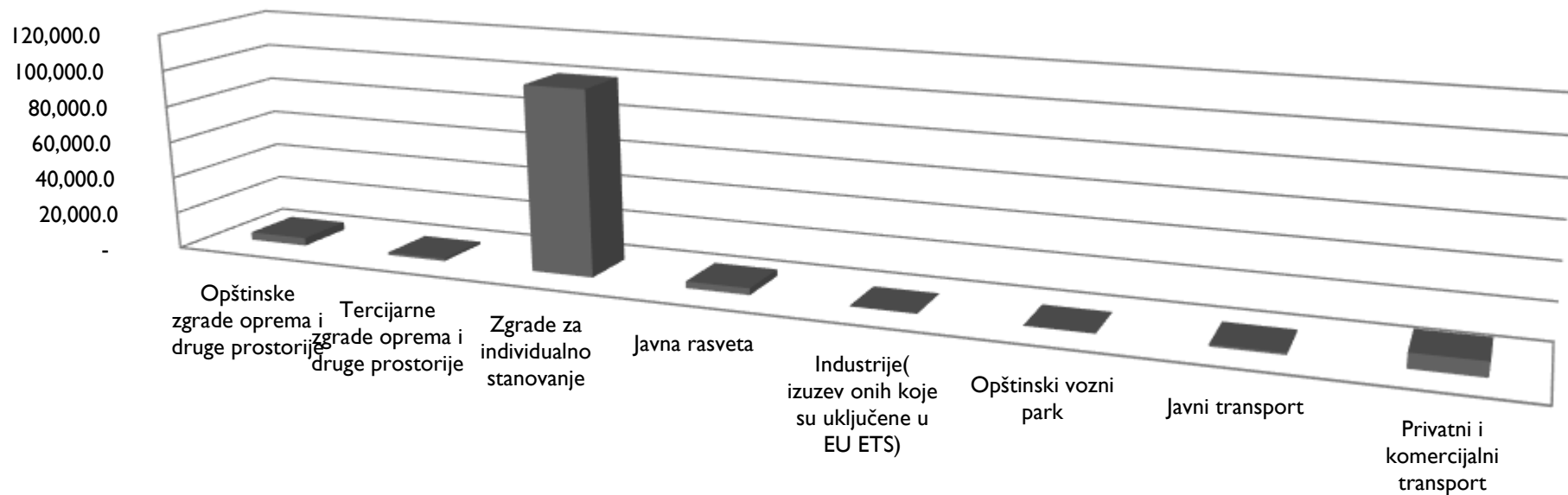
Emisije CO 2 po sektorima- Vrbas (tCO 2 godišnje)
